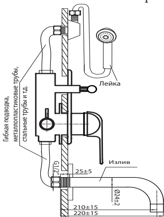
Возможные варианты установки и использования. Схема №2. Вар. №1
